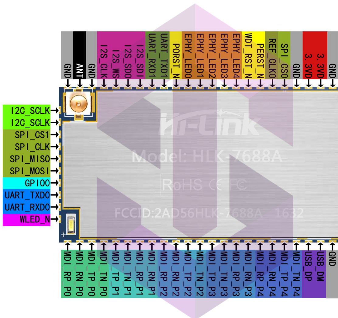
HLK-7688A 默认引脚定义图
